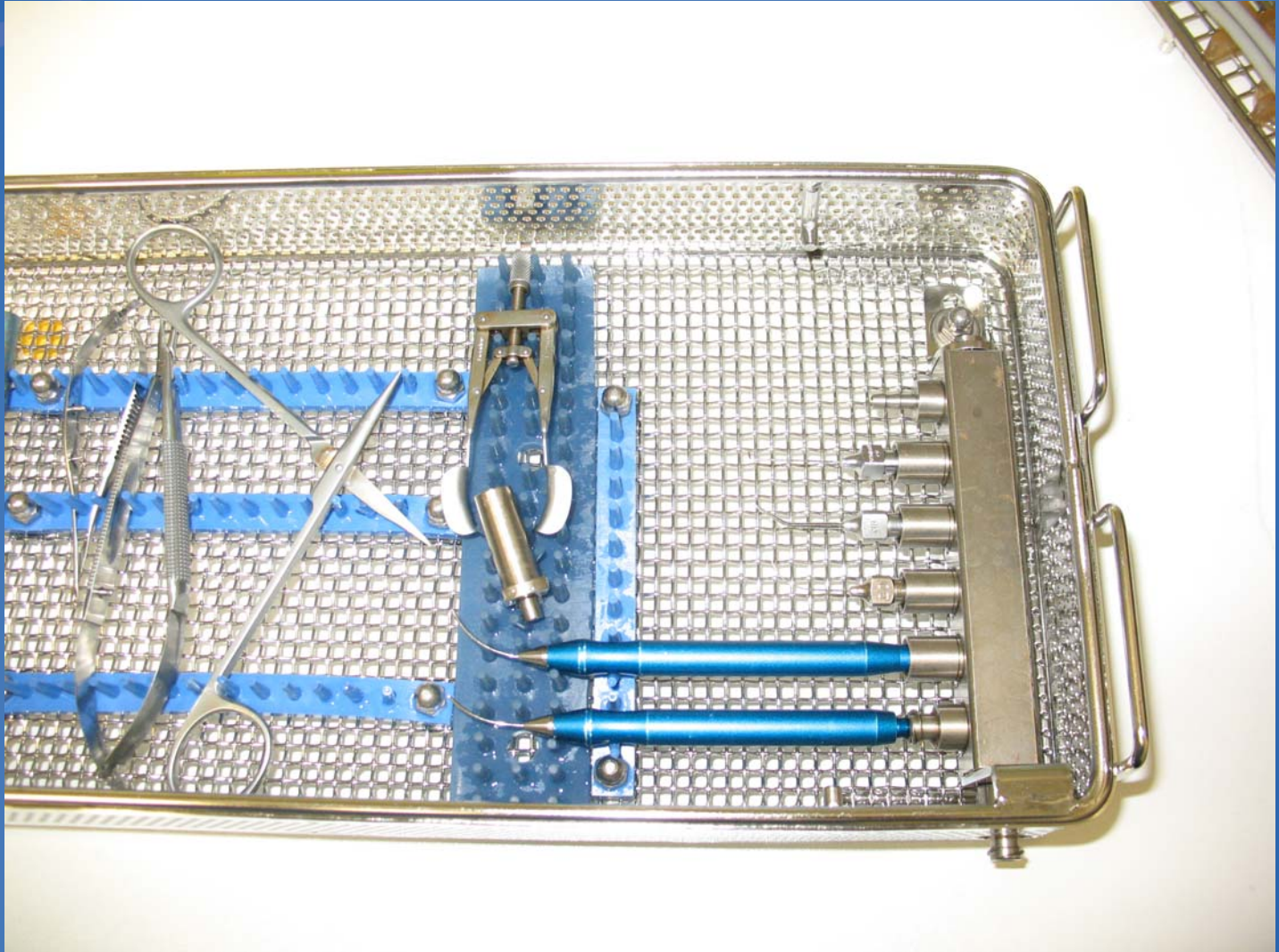
Katarakt Sieb - Ebene 1 mit zentralem Wasseranschluss
